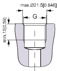
A: G main ports G: ISO 228/1 - G½
